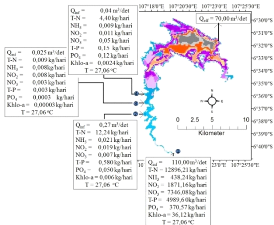
(b) Sebaran jumlah lapisan badan air, beban influen sungai dan debit efluen pada EMA 95 m
