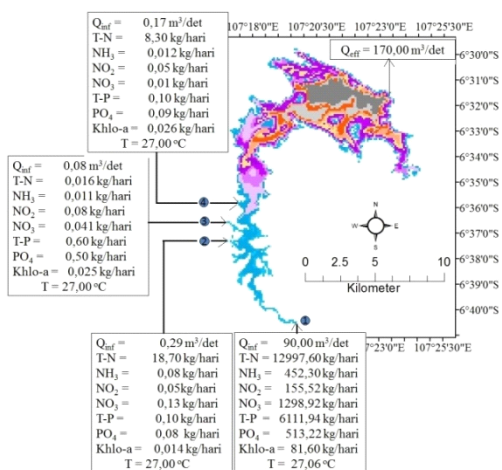
(c) Sebaran jumlah lapisan badan air, beban influen sungai dan debit efluen pada EMA 95 m
