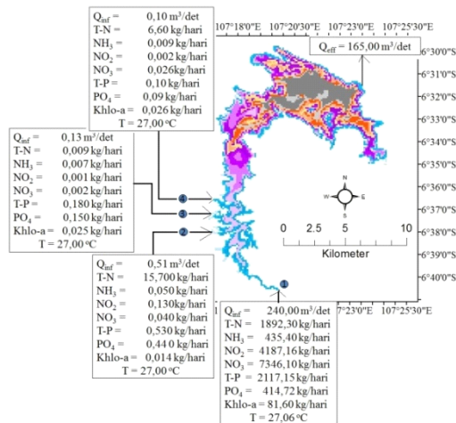
(d) Sebaran jumlah lapisan badan air, beban influen sungai dan debit influen sungai
