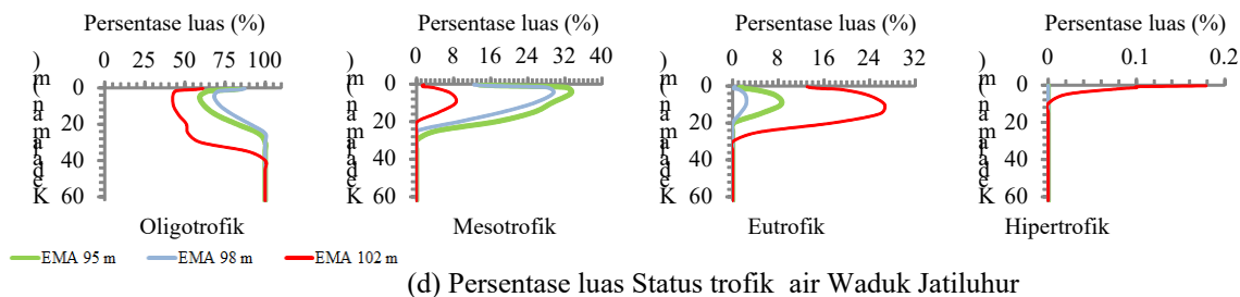
Gambar 7. Persentase luas status trofik dari sebaran spasial konsentrasi khlorofil-a di air Waduk Jatiluhur
