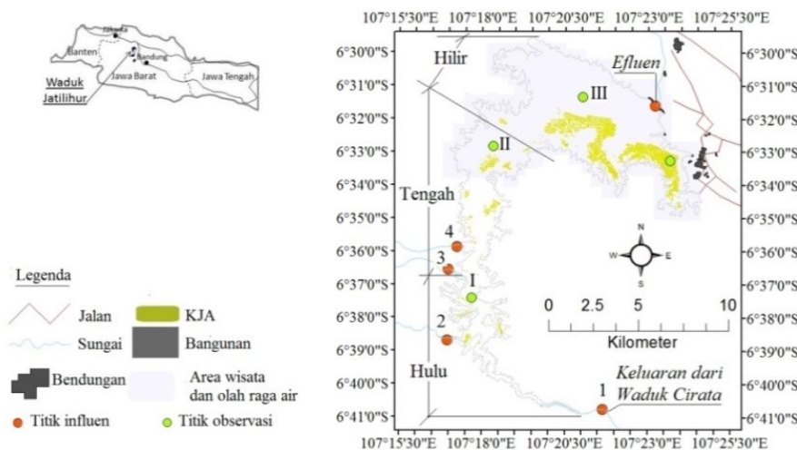
Gambar 1. Situasi perairan Waduk Jatiluhur
