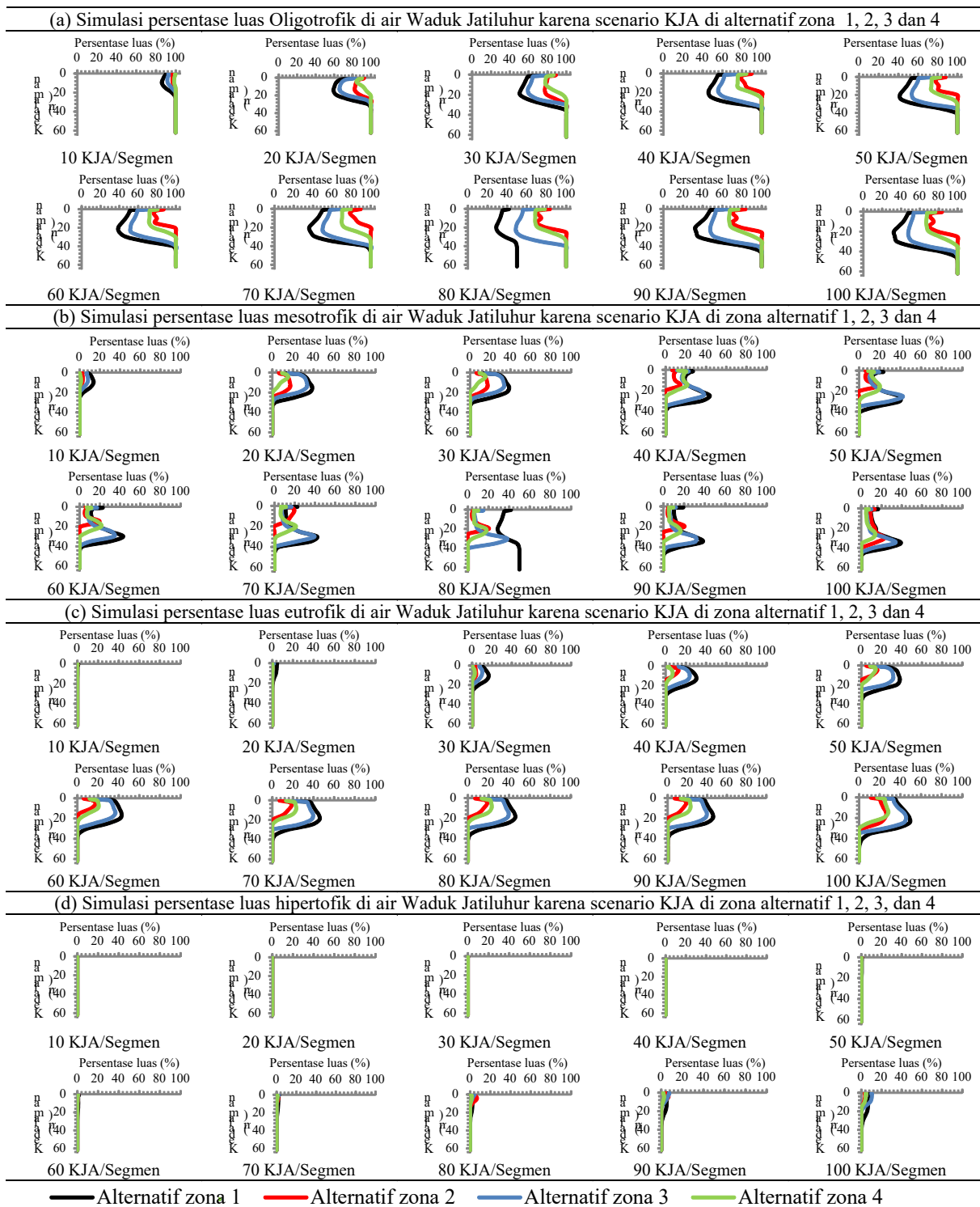
Gambar 8. Simulasi persentase luas status dari skenario budidaya ikan KJA di alternatif zona air Waduk Jatiluhur
