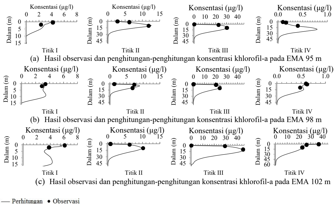
Gambar 5. Hasil observasi dan penghitungan-penghitungan model konsentrasi khlorofil-a di titik-titik stasiun observasi
